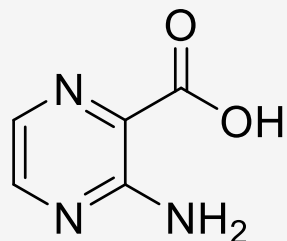
2-Amino-3-Carboxypyrazine
