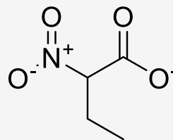
2-nitrobutanoate
