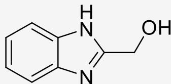
2-Benzimidazolemethanol
