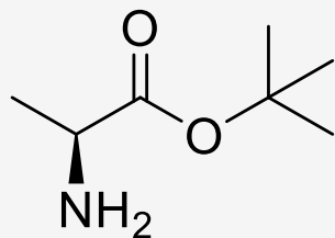
tert-butyl L-alaninate
