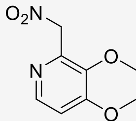
3,4-dimethoxy-2-(nitromethyl)pyridine
